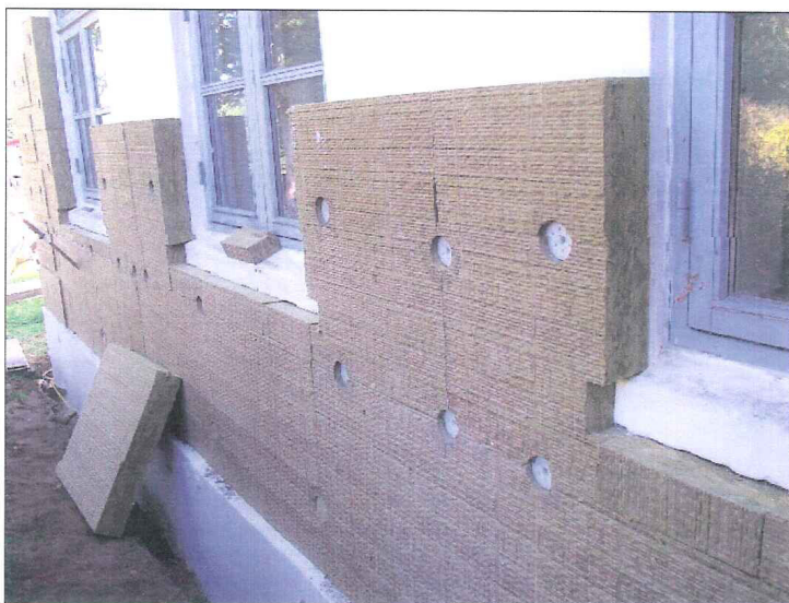
Et eksempel på energirenovering. Her er det Udviklingshøjskolen i Harte, der får efterisoleret. Oven på isoleringsbatsene bliver der påført et armeringsvæv, hvorefter facaden pudses op.
